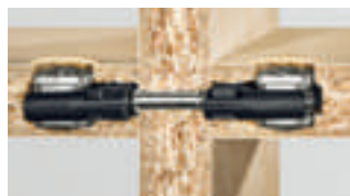
Spojky stredových strán – pre spoj DOMINO/LR 32
